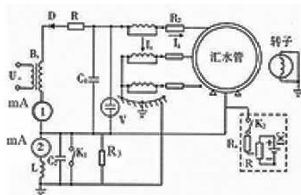
图一 直流试验低压屏蔽法接线
