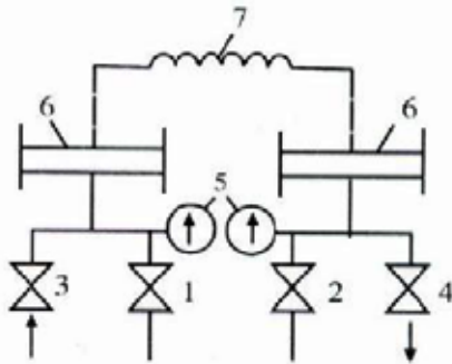
图2 “充水” 示意图
