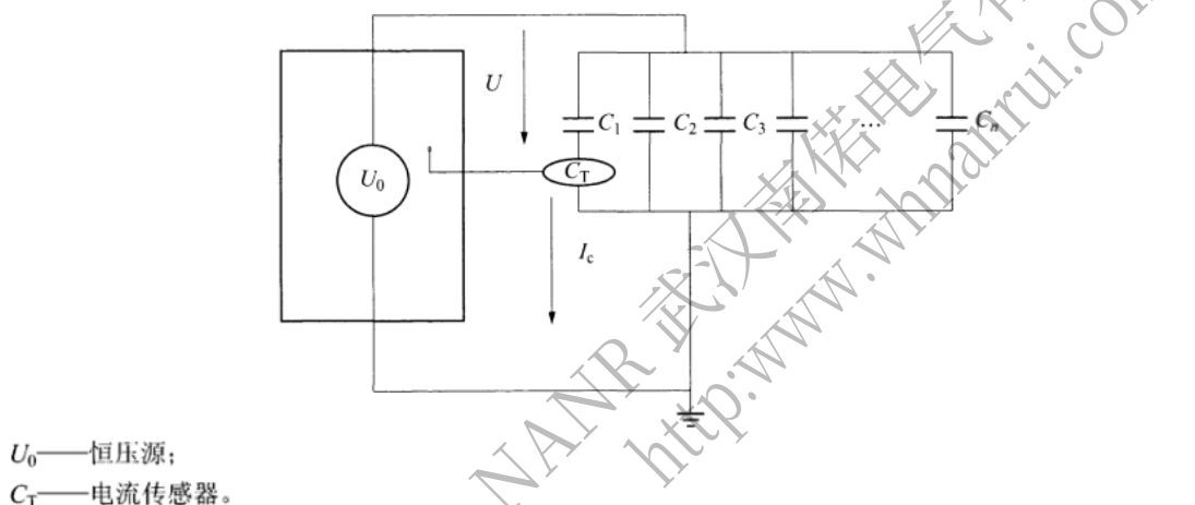
图 1 测试仪测量电力电容器接线图
