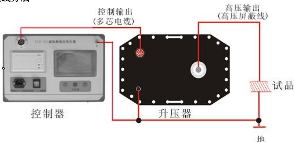
图4 (连线图)
