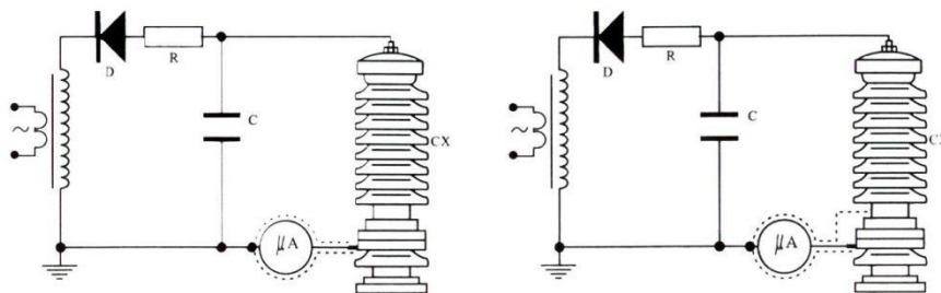
微安表接入试品CX底部的接线图
