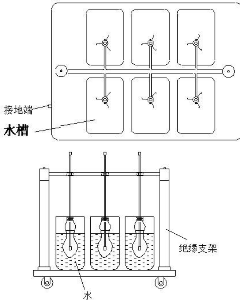
图 3-2 绝缘靴（手套）试验台
