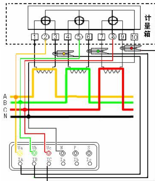
三相电路接线示意图
