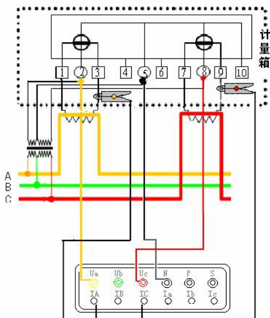
三相三线电路接线示意图
