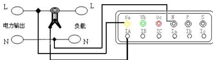
单相电路接线示意图
