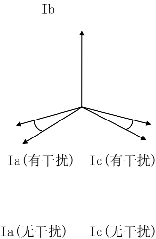
图十三、AC 相受 B 相影响
