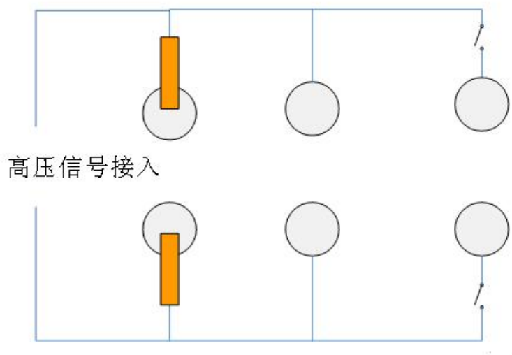
图 2 分合终端原理图
