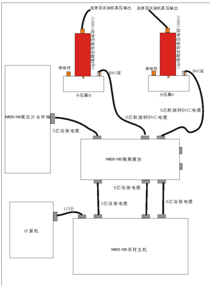
图 3 测试系统连线图
