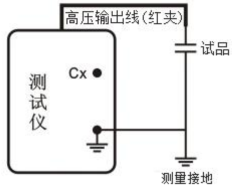
图 12 反接法
