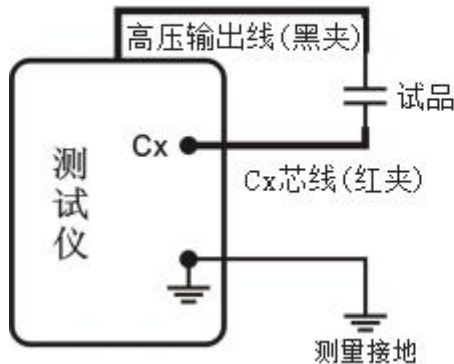
图 11 正接法
