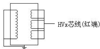
图8 PT接法
