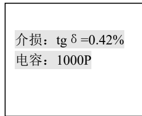
图 9 测量结果
