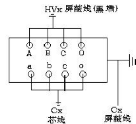
图12 变压器接法
