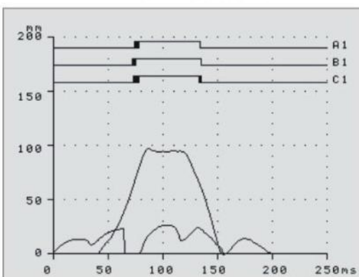
合--分闸测试图形
