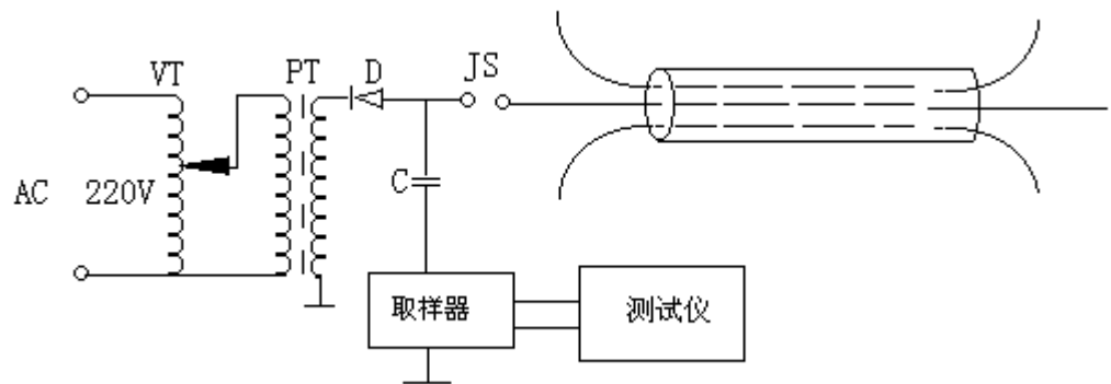
图 6.4-1 电流取样法测试线路
