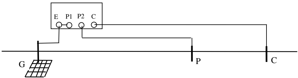
G 一被试接地装置 C 一电流极 P—电位 图 2 接地电阻测试接线示意图
