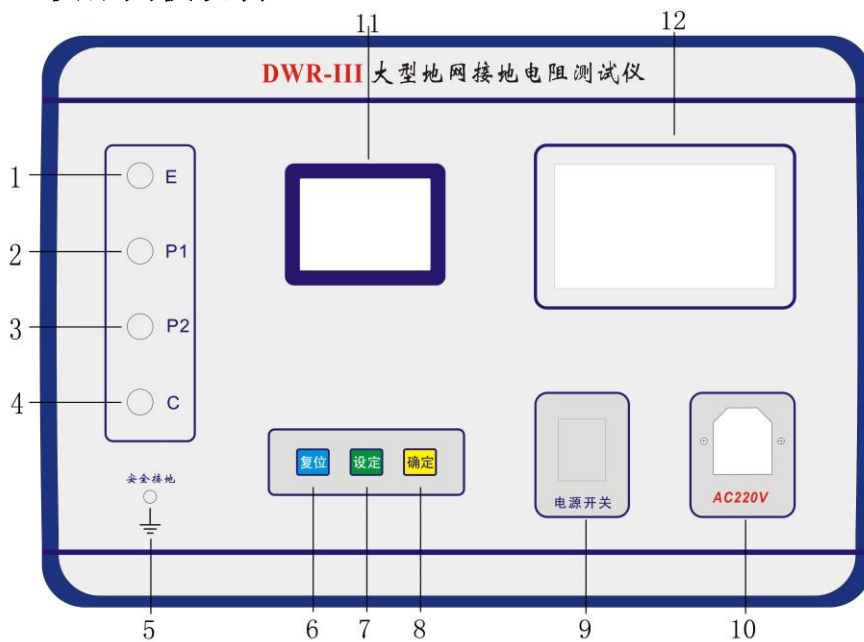
仪器面板布置图
