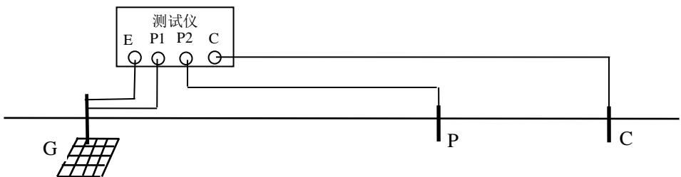
G 一被试接地装置 C 一电流极 P—电位 图 3 接地阻抗测试接线示意图
