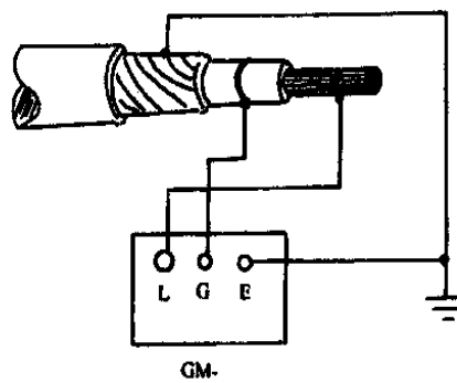
屏蔽电缆绝缘测试接线图
