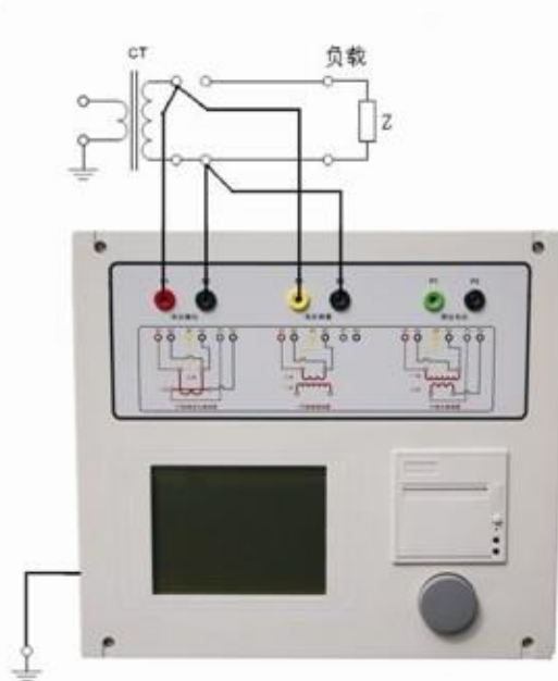
图 2.2 CT 二次负荷试验接线方式
