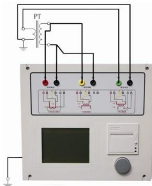
图 2.8 PT 变比、极性试验接线方式
