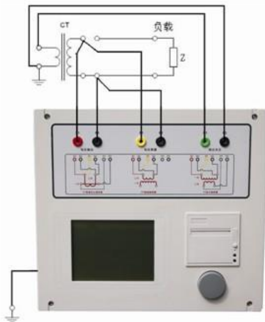
图 2.1 CT 直阻、励磁、变比试验接线方式
