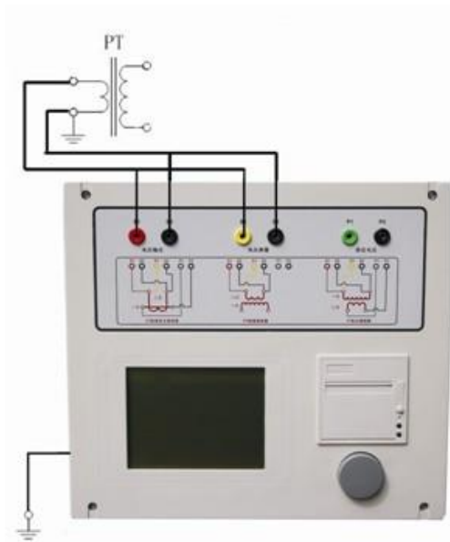
图 2.7 PT 直阻、励磁试验接线方式
