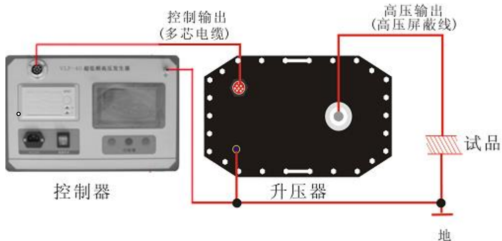
图4 (连线图)
