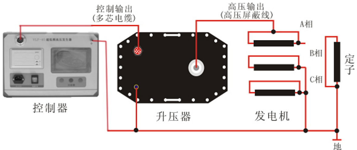
图 14 测量定子的某相连线图
