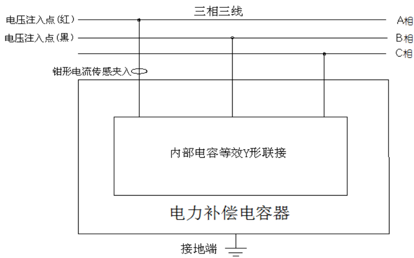
Y 形联接被试电容 AB 相接线图
