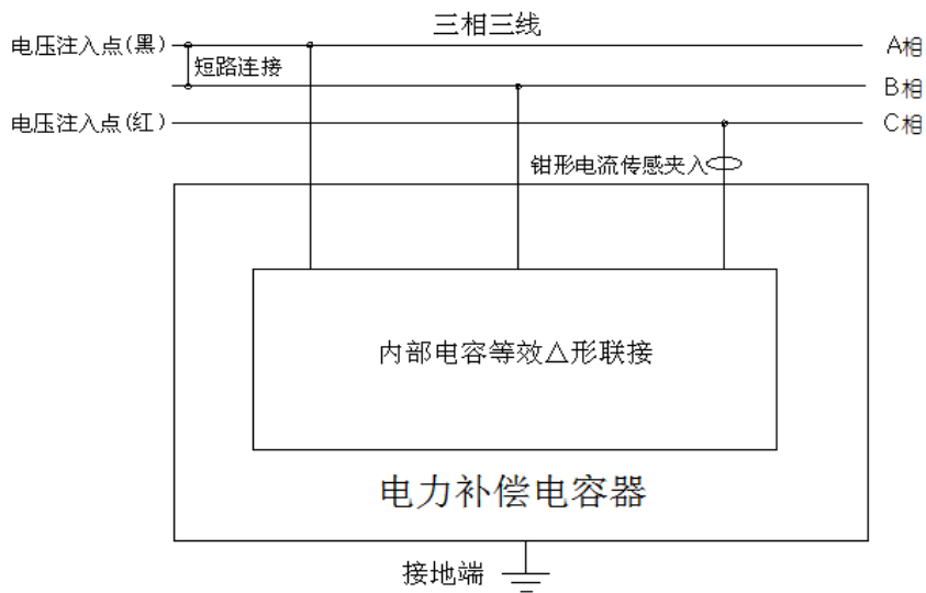
△形联接被试电容 CA 相接线图
