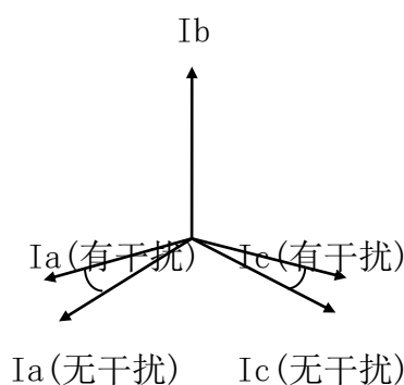
图十三、AC 相受 B 相影响
