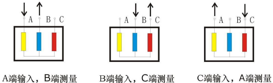
图 4.1.2 Y 接线
