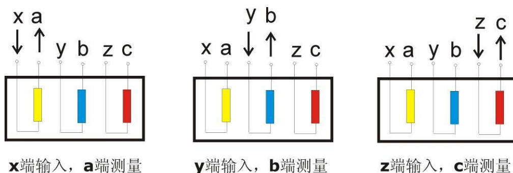
图 4.1.4 外连接 \Delta 接线
