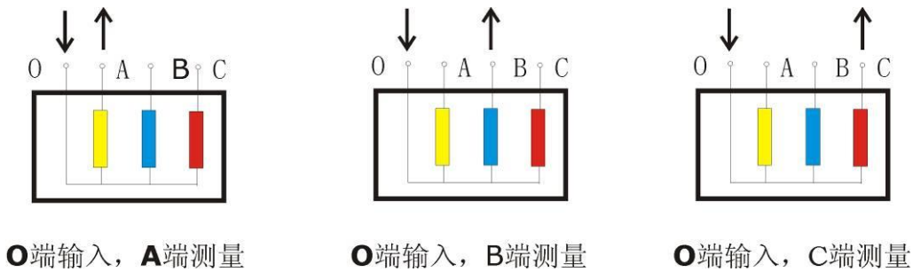
图 4.1.1 YN 接线
