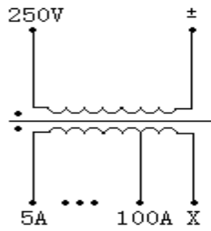
三、电流互感器自校线路图
