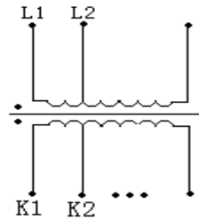
四、电流互感器检定线路图
