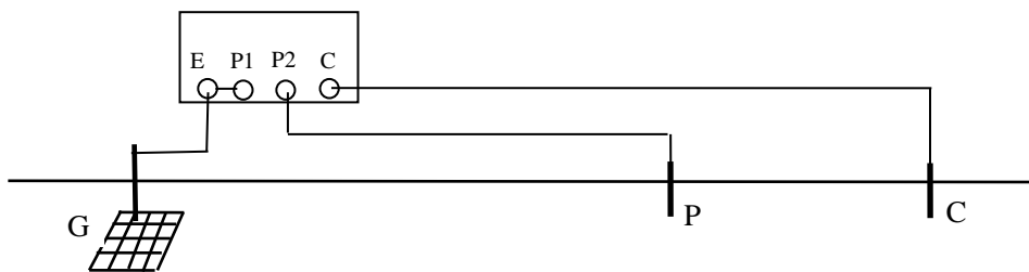
G —被试接地装置 C —电流极 P—电位 图 2 接地电阻测试接线示意图
