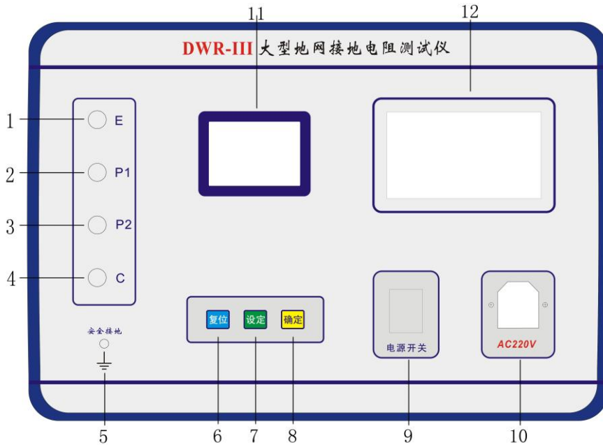
仪器面板布置图
