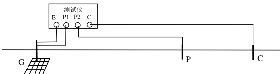
G —被试接地装置 C —电流极 P—电位 图 3 接地阻抗测试接线示意图
