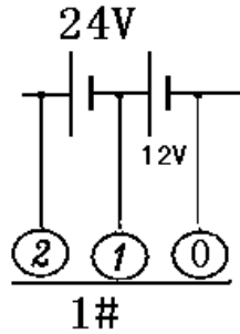
12V 或者 6V 单个数据采集盒接线图
