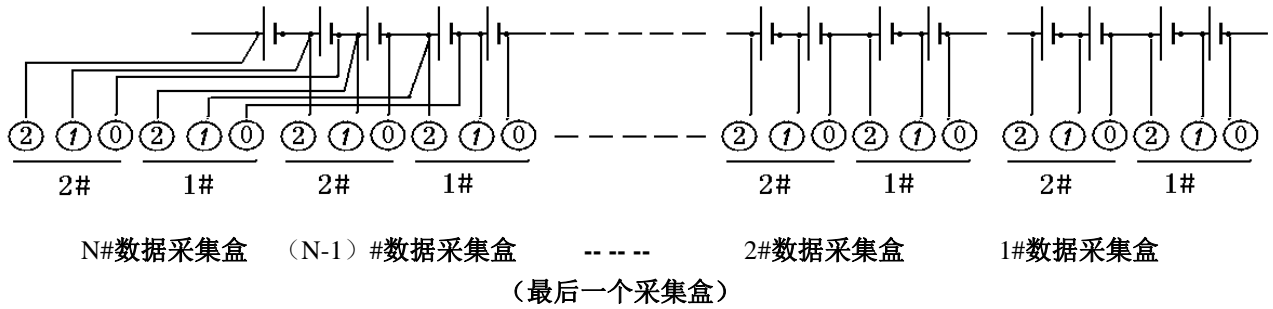
电池数量有多余时采集盒接线图.
