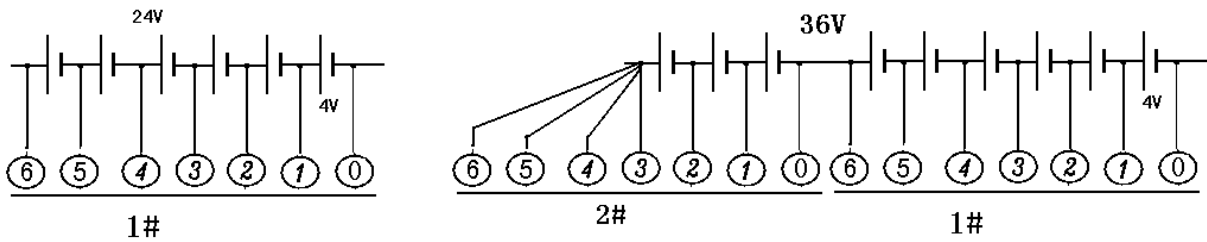
电池数少于一个采集盒能采集的相应电池数时接线图
