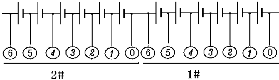
2V 或者 4V 单个数据采集盒接线图
