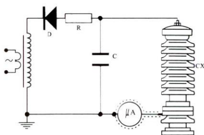
微安表接入试品CX底部的接线图
