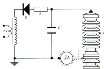
排除试品CX表面影响接线图
