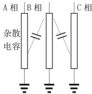
图九、一字排列避雷器
