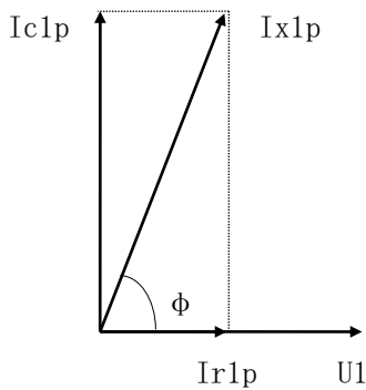
图八、投影法
