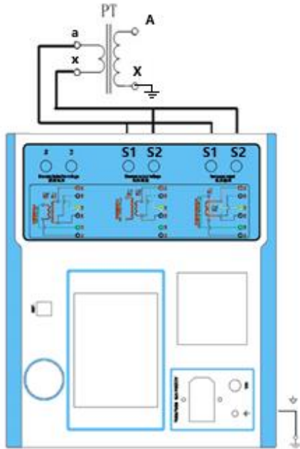
图 2.7 PT 直阻、励磁试验接线方式
