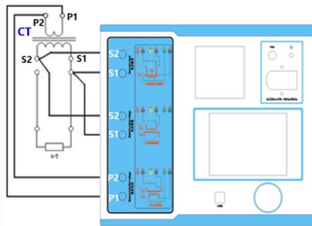
图 2.1 CT 直阻、励磁、变比试验接线方式
