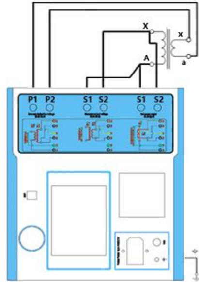
图 2.8 PT 变比、极性试验接线方式
