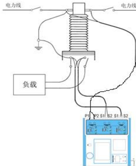
图 C.1 典型接线方式
